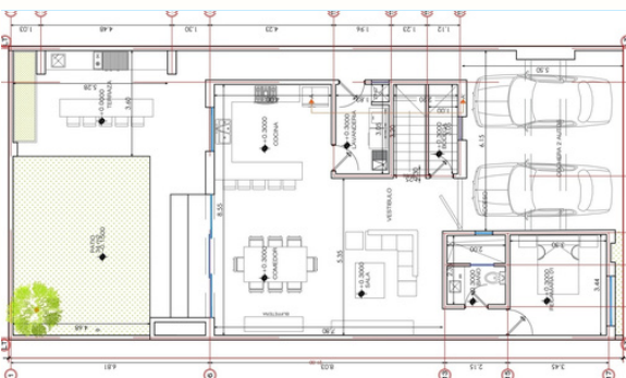
PLANTA BAJA
